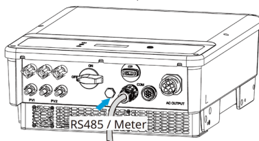
AS-IC02-8000-2 | AS-IC02-10000-2
